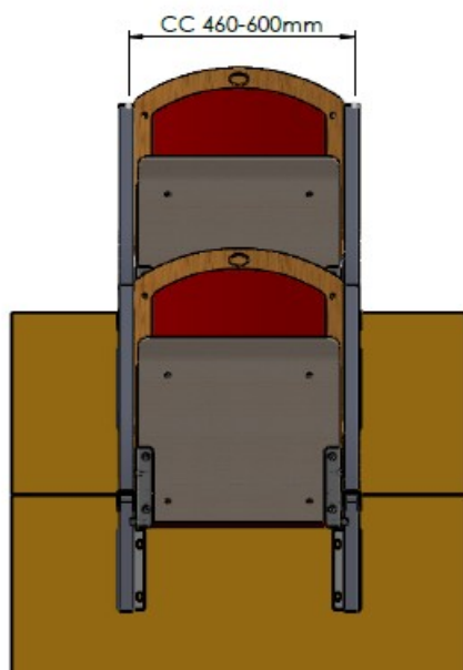
C/C 460 - 600 mm
