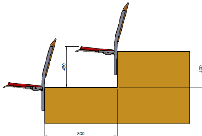
Stadion Comfort med motvikt måttskiss för 450 mm hög gradäng
