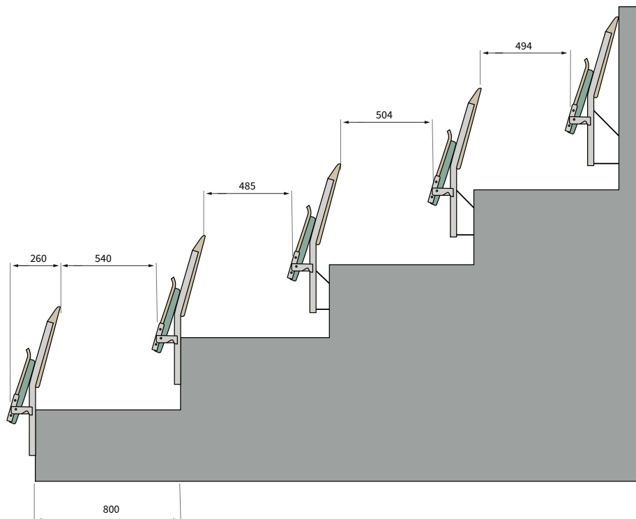
Stadion Comfort med dubbla fjädrar. Måttskissen är för 450 millimeter hög gradäng.
