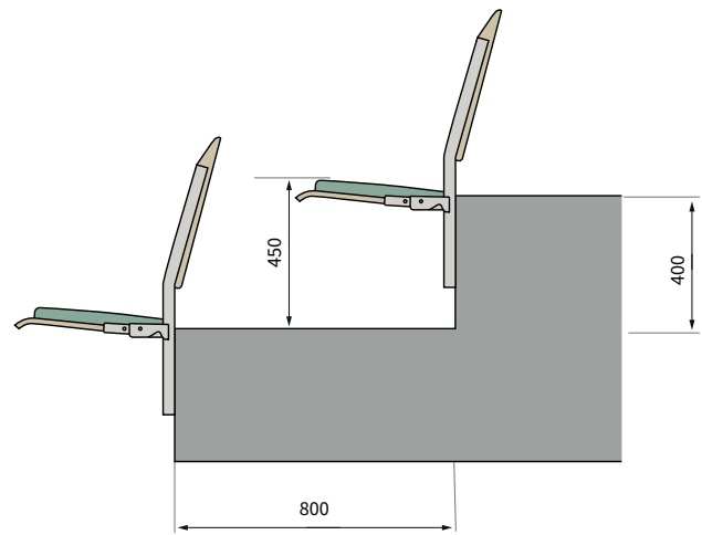
Stadion Comfort med motvikt. Måttskiss för 450 millimeter hög gradäng.
